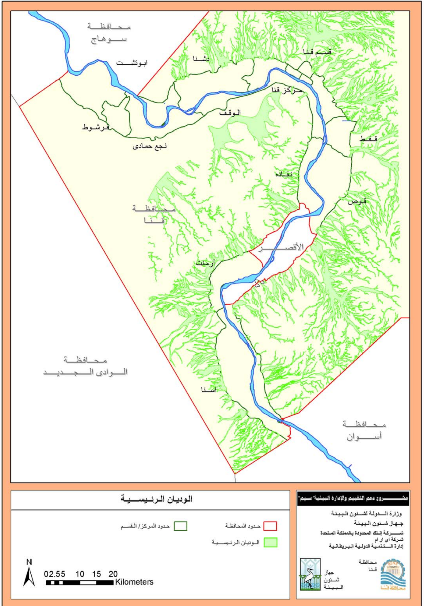
خريطة رقم (٩) الوديان الرئيسية بمحافظة قنا
